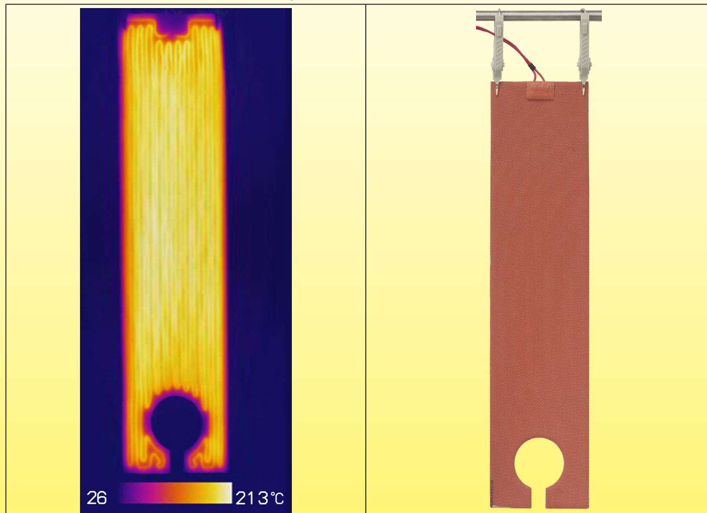
Imagen termográfica de una cinta calefactora de silicona plana de 2,4 mm con una carga de potencia superficial de 1 \text{ W}/\text{cm}^2 , suspendida en aire tranquilo, no fijada en una placa, a una temperatura ambiente de 25^\circ\text{C} . La temperatura superficial alcanza los 213^\circ\text{C} , cerca de su destrucción.
