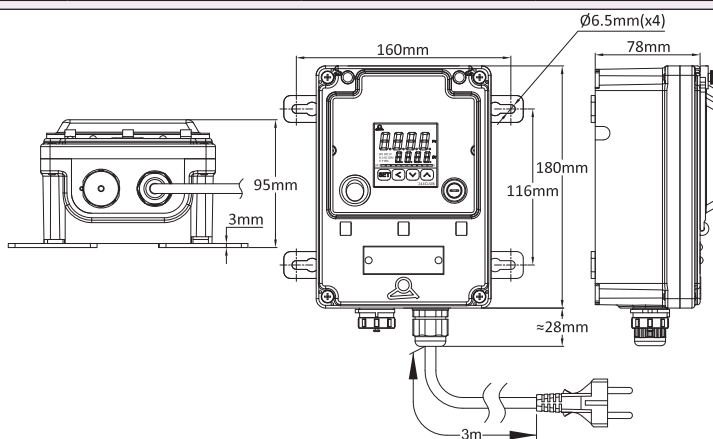
Modelo con conector impermeable de 5 vías
