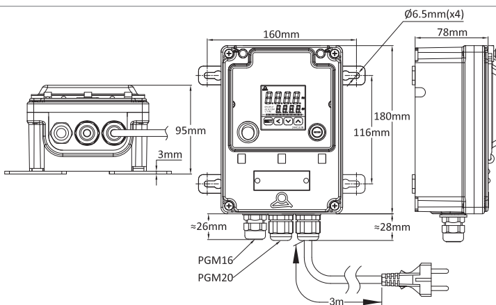
Modelo con 3 glándulas de cable
